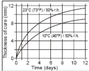
1. diagram: A Sikaflex®-527 AT térhálósodási sebessége
