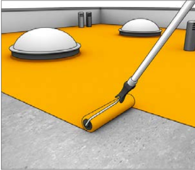
Sikalastic-580 felhordása hengerrel.
